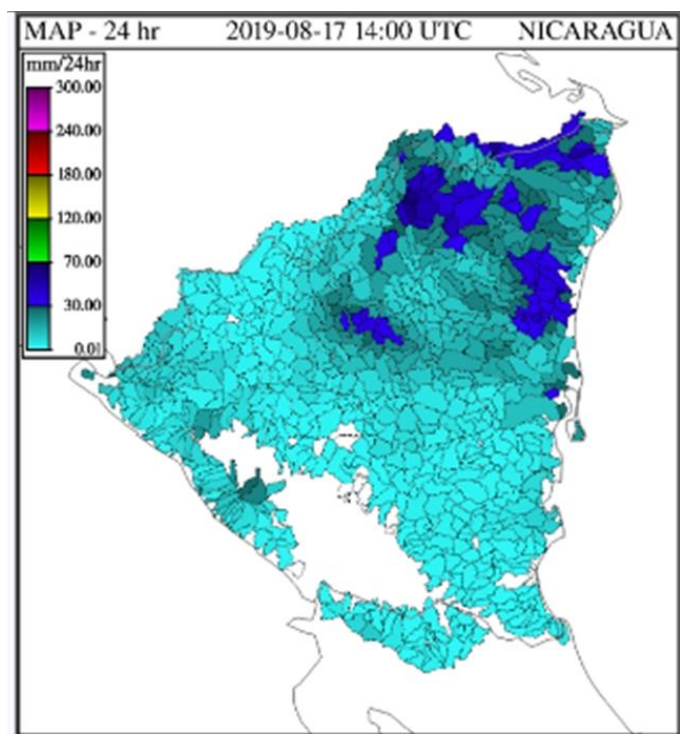
Precipitación acumuladas en las ultimas 24 horas
