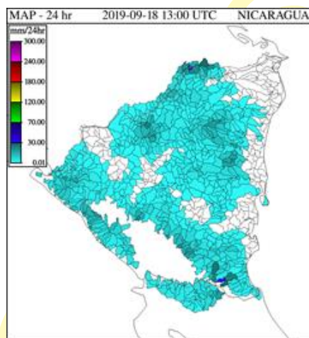
Precipitación Acumulada en 24 horas
