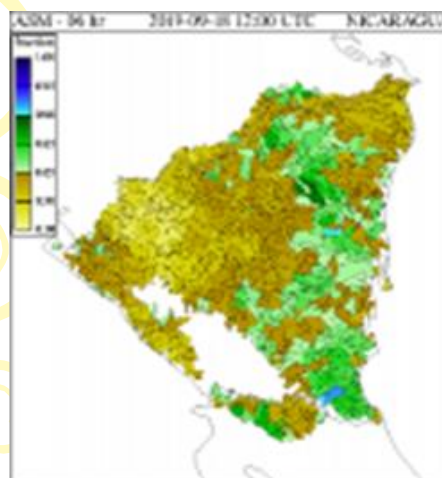
Grado de Saturación del Suelo (%)
